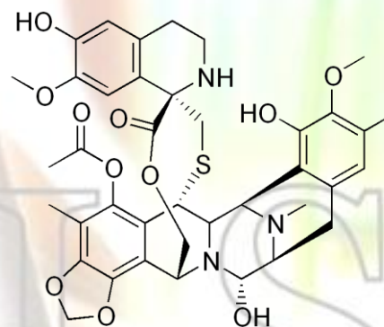
Trabectedin
